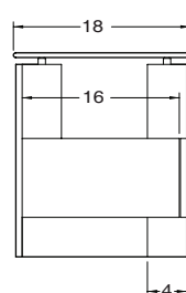
VUE DE CÔTÉ / SIDE VIEW
