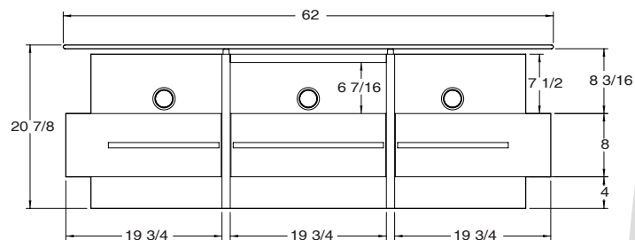
VUE DE FACE / FRONT VIEW
