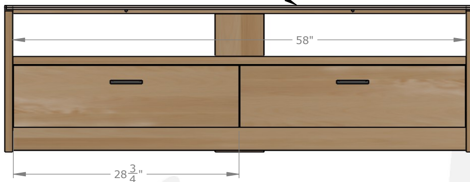
MEUBLE AUDIO-VIDÉO / TV STAND 18 x 60 x H 19 CONDO BTM 1860
